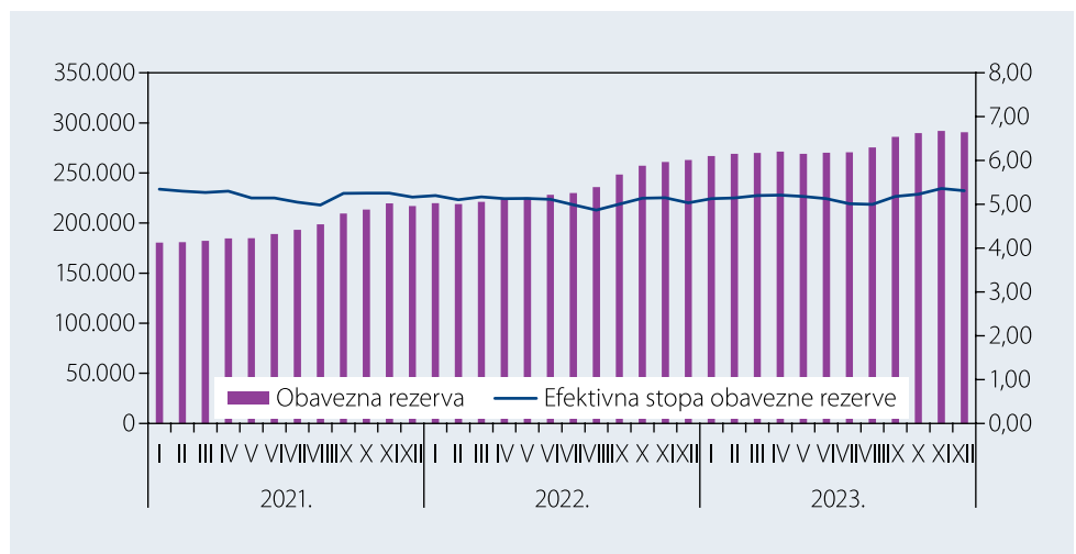
Grafikon 7 – Izdvojena obavezna rezerva u 000 eura (lijeva skala), efektivna stopa obavezne rezerve, u % (desna skala), januar 2021 - decembar 2023, stanje na kraju mjeseca
